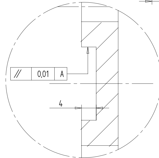
Détail B 2:1
