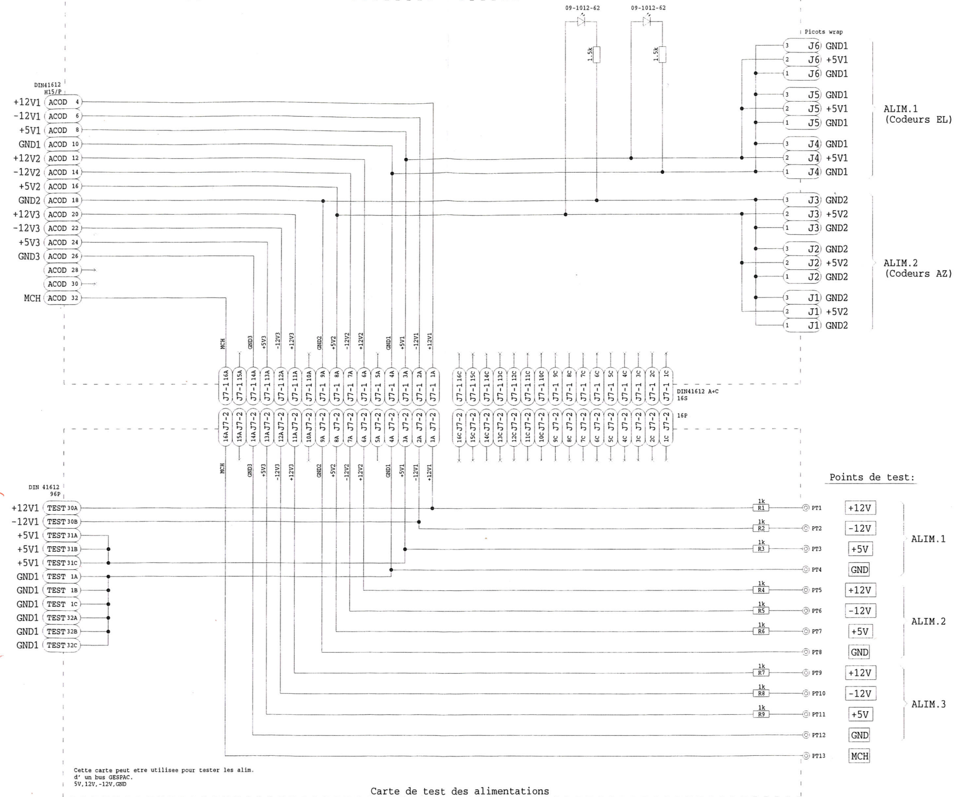
Carte de test des alimentations
