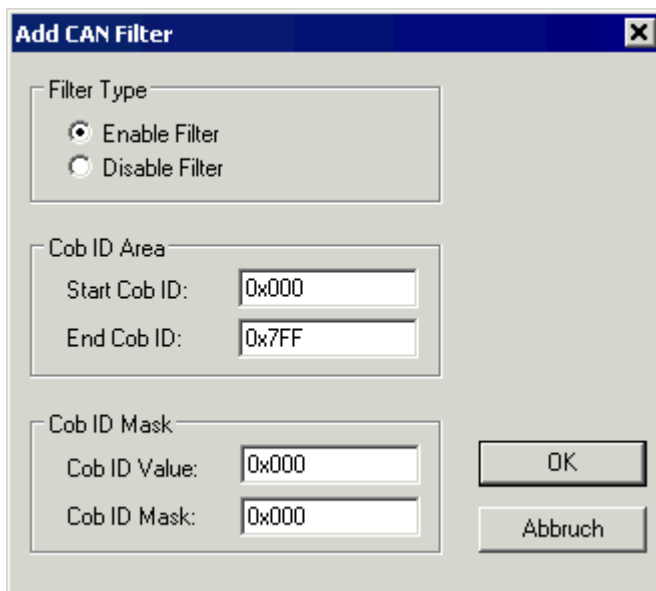
Fig. 97: Dialog „Add CAN Filter“
