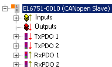
Fig. 100: EL6751-0010 TwinCAT tree
