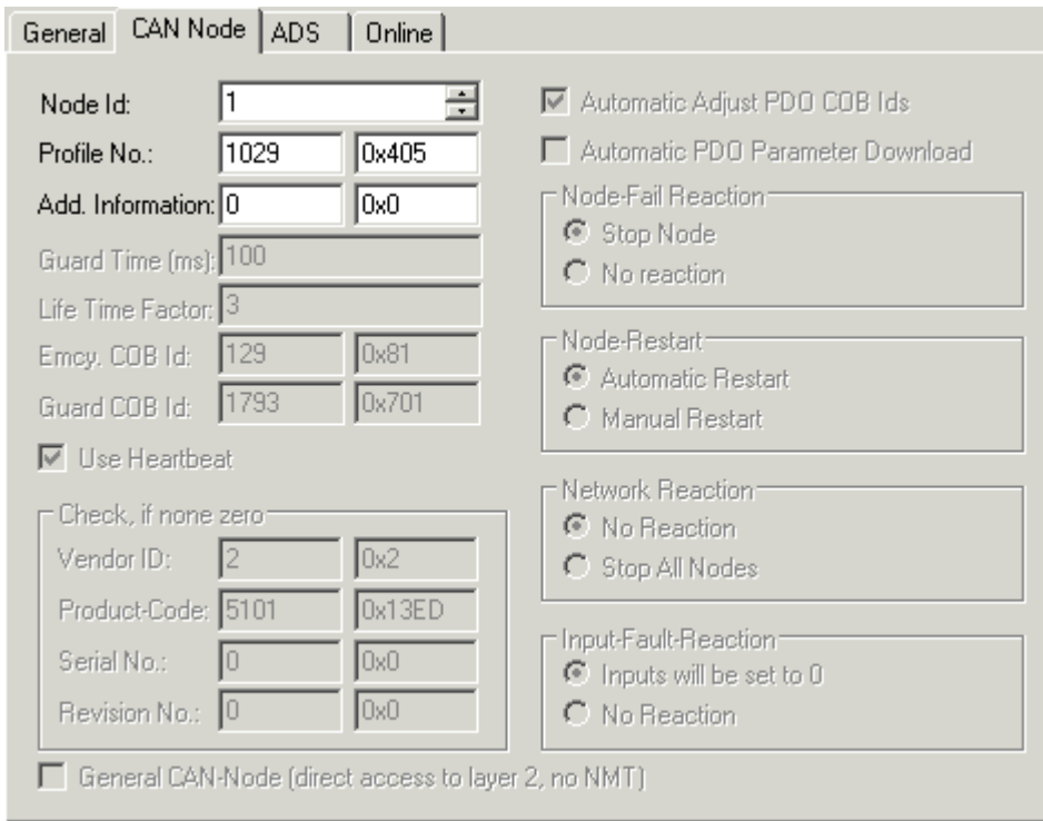
Fig. 101: "CAN node" tab
